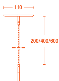
Hängevorrichtung
