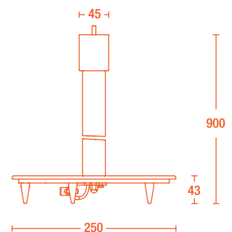
Standfuß
